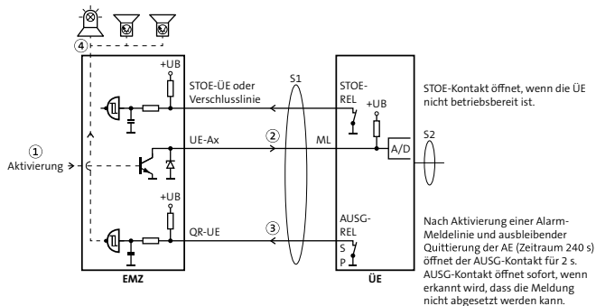
Funktion mit Negativquittung anhand Beispiel mit paralleler Anschaltung
