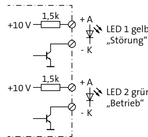
LED-Ausgänge „Störung“ und „Betrieb“
